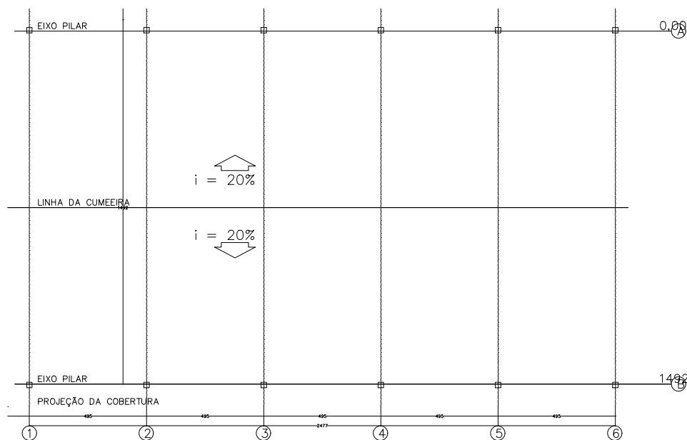
PLANTA BAIXA Escala 1 : 50 Medidas em "cm"
