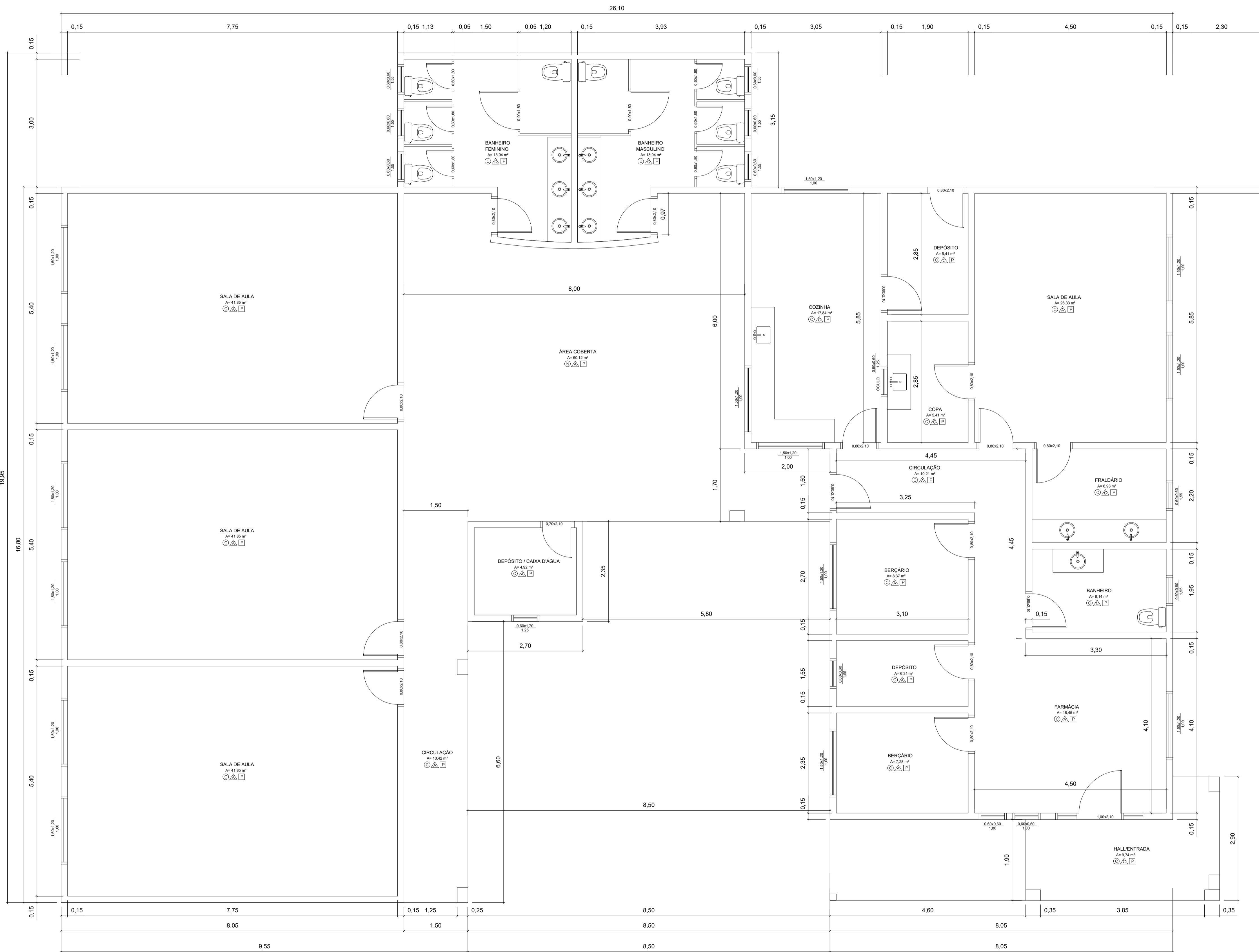
PLANTA BAIXA ESC 1:100 ÁREA: 389,29m 2
