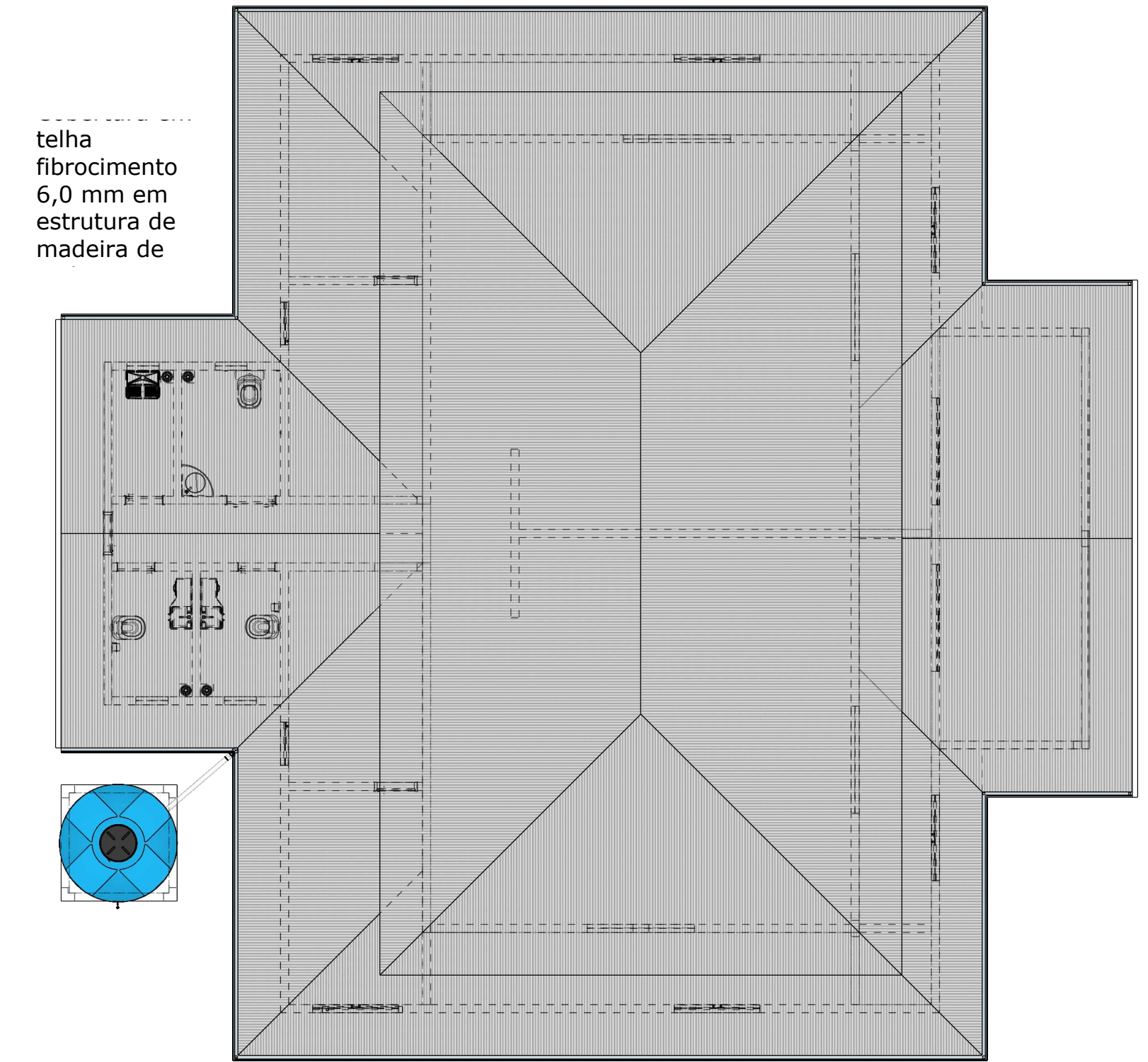
A 02 PLANTA BAIXA COBERTURA ESCALA _____ 1/100
