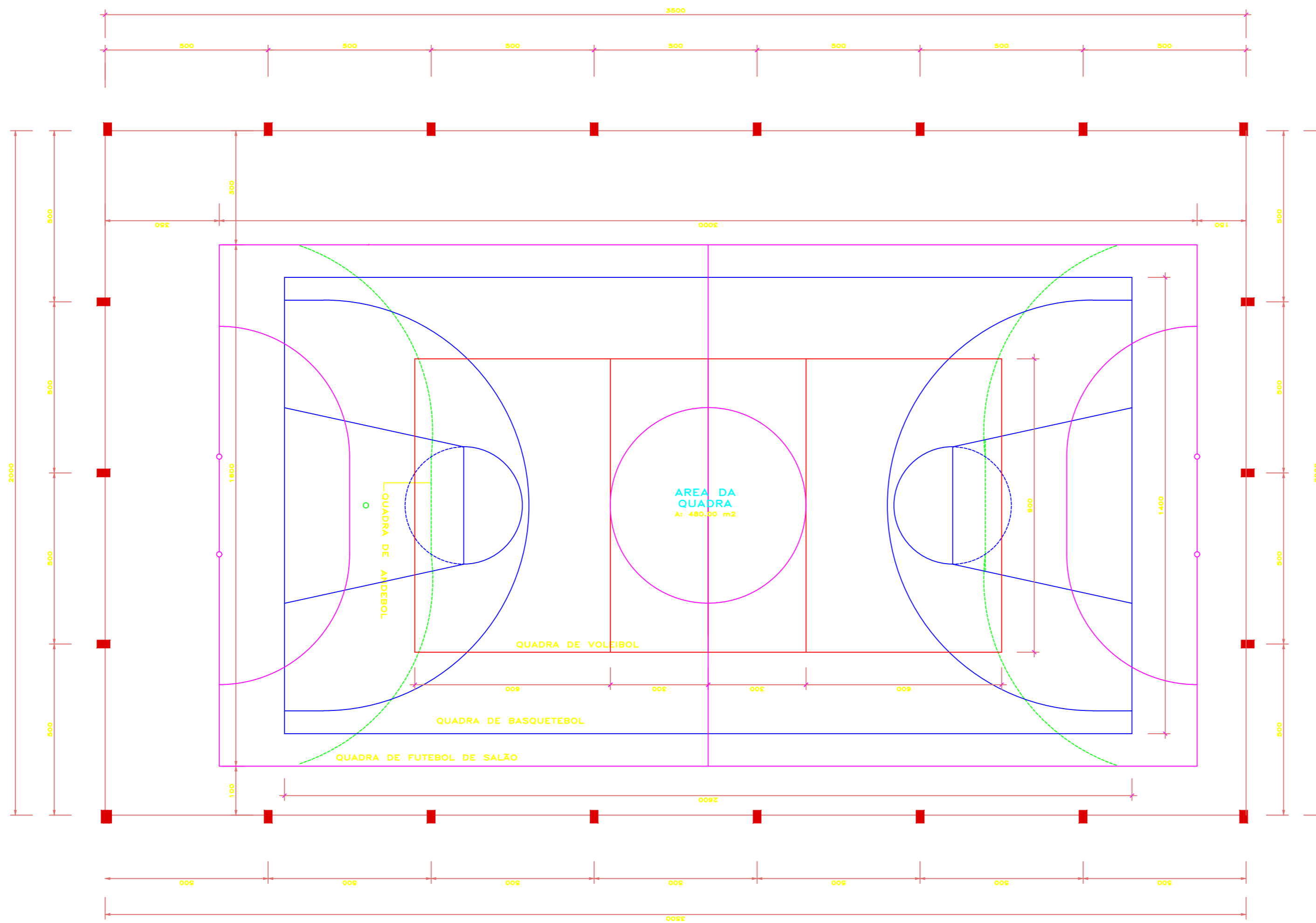
PLANTA BAIXA ESC. 1 / 75 AREA=700,00m2
