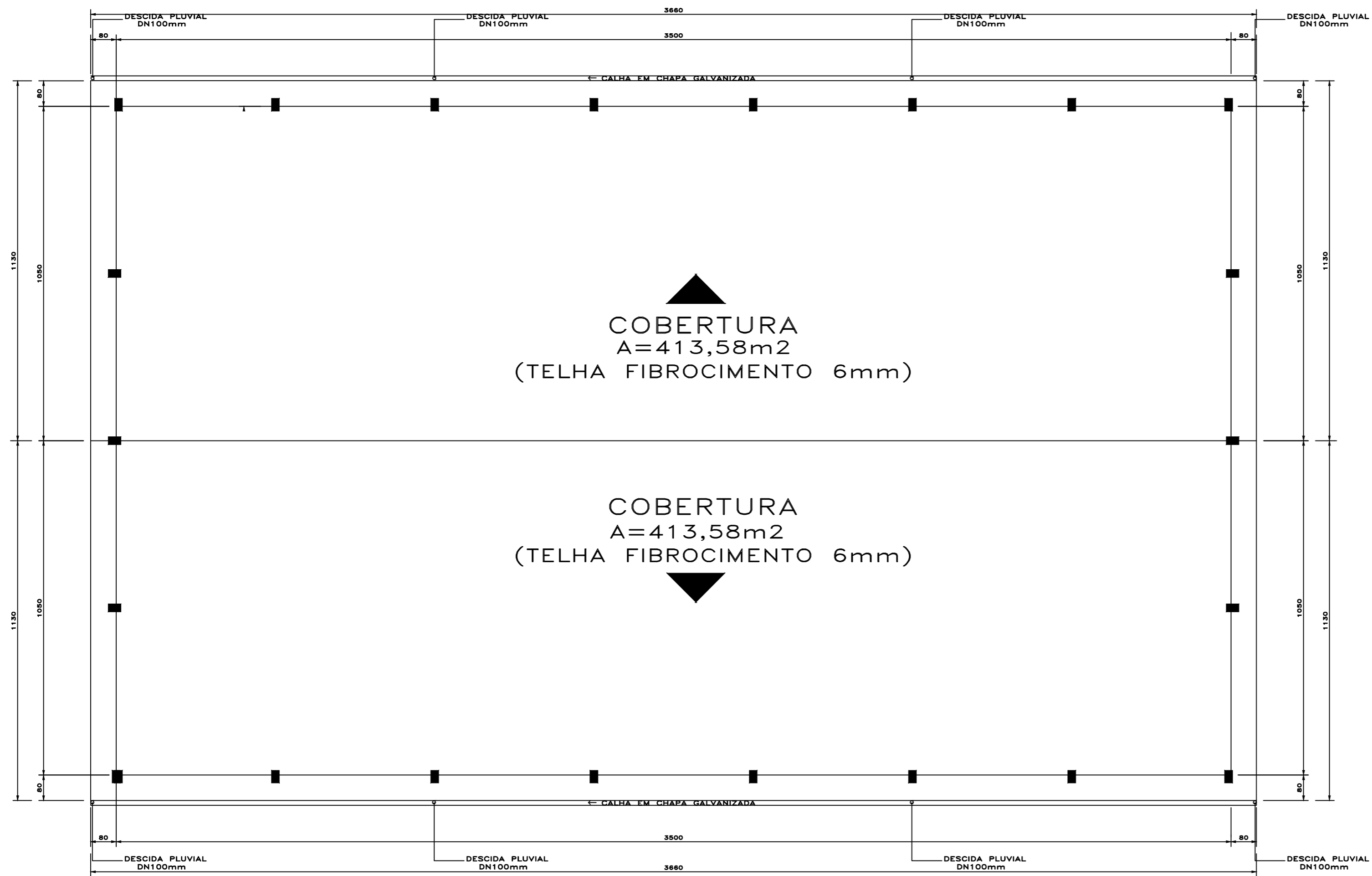
PLANTA DE COBERTURA CAPTAÇÃO ÁGUAS PLUVIAIS ESC. 1 / 75
