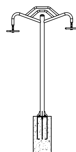
DETALHE EQUIPAMENTO ALONGADOR DUPLO EM VISTA
