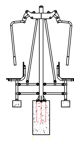
DETALHE EQUIPAMENTO PUXADOR COSTA DUPLO EM VISTA E FUNDAÇÃO
