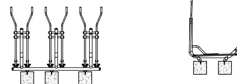
DETALHE EQUIPAMENTO ESQUI TRIPLO EM VISTA FRONTAL E LATERAL
