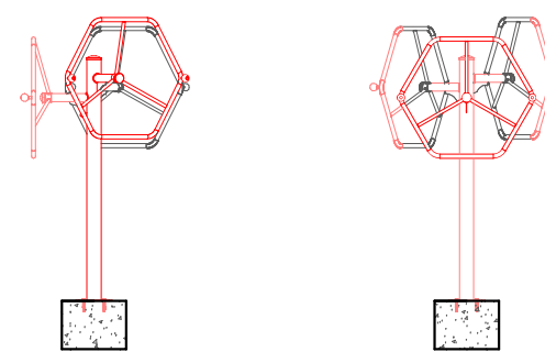
DETALHE EQUIPAMENTO ROTAÇÃO VERTICAL TRIPLO- VISTA LATERAL E FRONTAL
