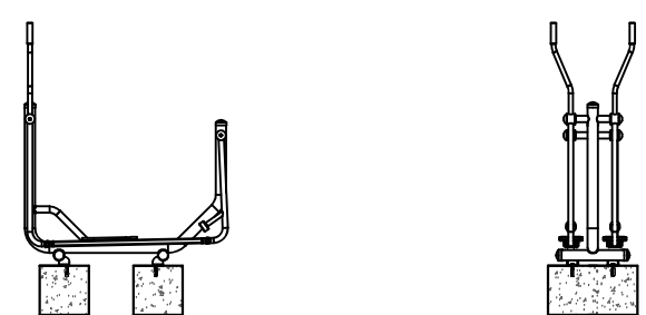
DETALHE EQUIPAMENTO ESQUI INDIVIDUAL EM VISTA
