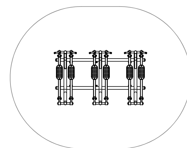
DETALHE EQUIPAMENTO ESQUI TRIPLO PLANTA BAIXA
